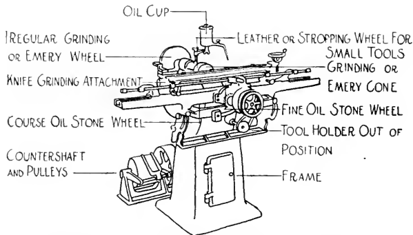
FIG. 217. AUTOMATIC KNIFE GRINDER.
